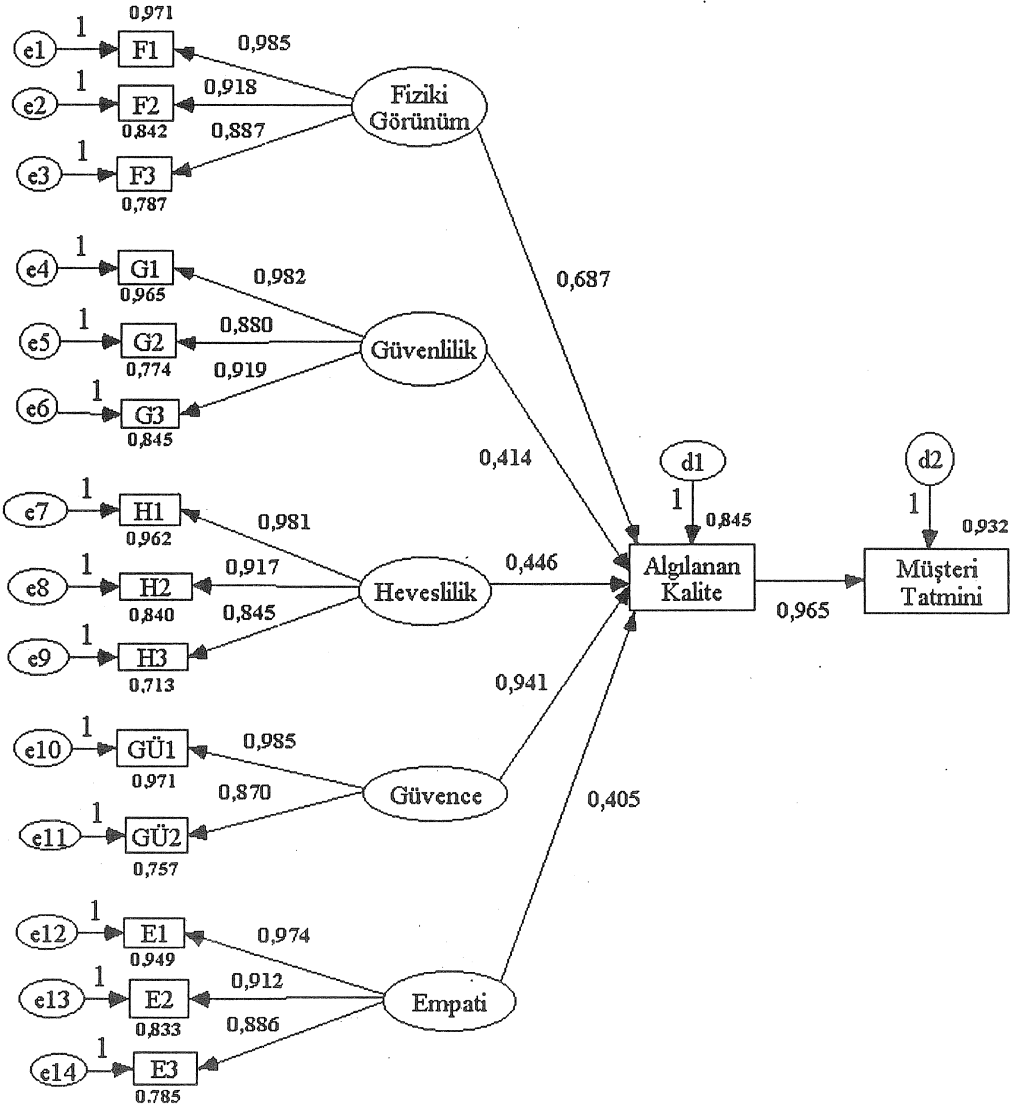
Şekil 2. Araştırma Modeli Testinin AMOS çıktısı
