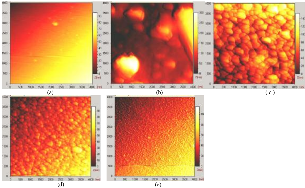
Fig 3. AFM images(4 \mu m \times 4 \mu m) of ZnO thin films. (a) %5 O 2 + %95 Ar (b) %10 O 2 + %90 Ar (c) %15 O 2 + %85 Ar (d) %20 O 2 + %80 Ar (e) %30 O 2 + %70 Ar.
