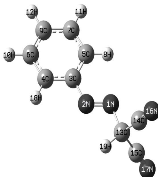
Azo
