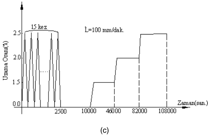
Şekil 2. a) Direkt prosedür, b) Normal prosedür, c) Ön prosedür uygulanmış gerilme gevşemesi deney prosedürleri
