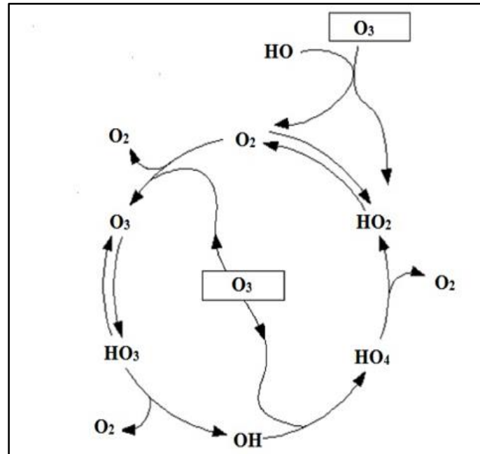
Şekil 2. Sudaki O_3 'ün OH^- iyonu tarafından başlatılan bozunması için dairesel zincir mekanizması. [9,11].
